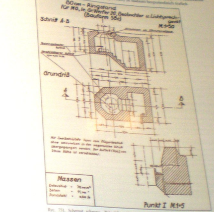
Ryc. 771. Schemat schronu „Tobek” według niemieckich rysunków technicznych – w zbiorze Włodzisława Gubowskiego
